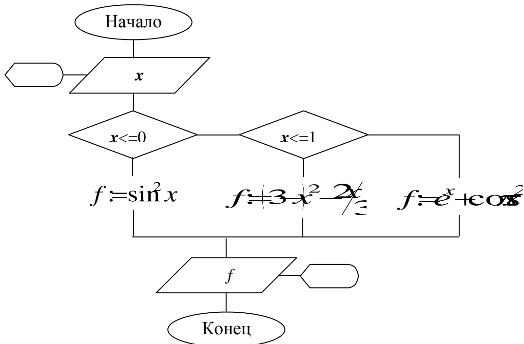
Рис. 20. Пример блок-схемы разветвляющегося алгоритма
