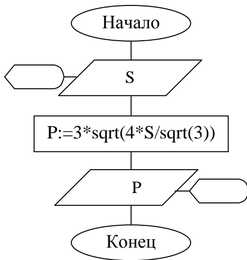
Рис. 19. Пример блок-схемы линейного алгоритма
