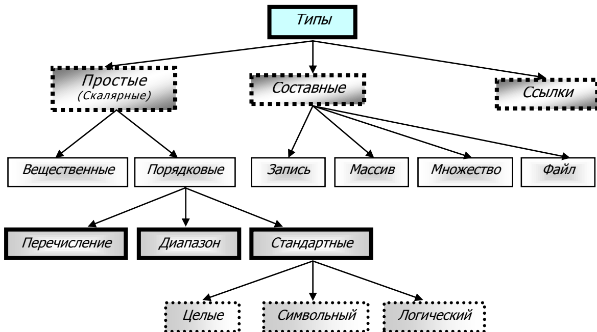
Рис. 17. Иерархия типов языка Паскаль
